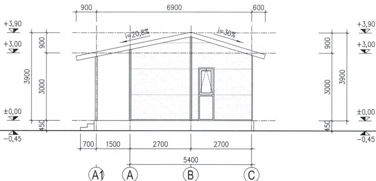
MẶT ĐÚNG BÊN (TỶ LỆ : 1/100)
